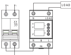
Рис. 8 Схема подключения
